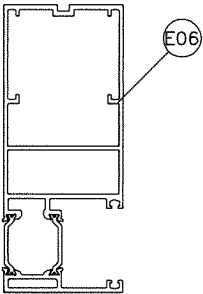
JAMB 'J'
