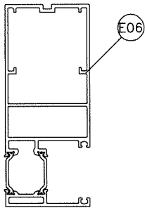
JAMB 'J'
